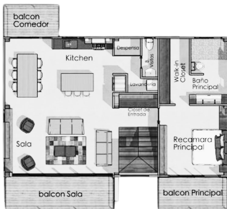
Nivel 03
